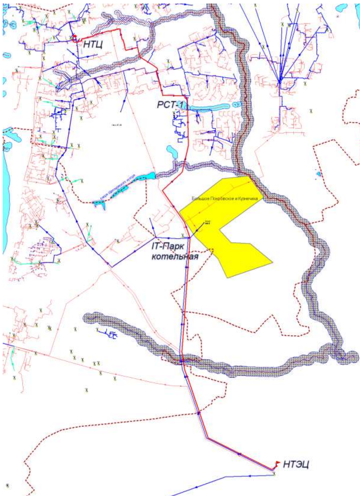
Рисунок 2.2 – Трасса от НГТЭЦ через котельную IT-Парка, через РСТ-1 по т/м «3 очередь» до НТЦ
